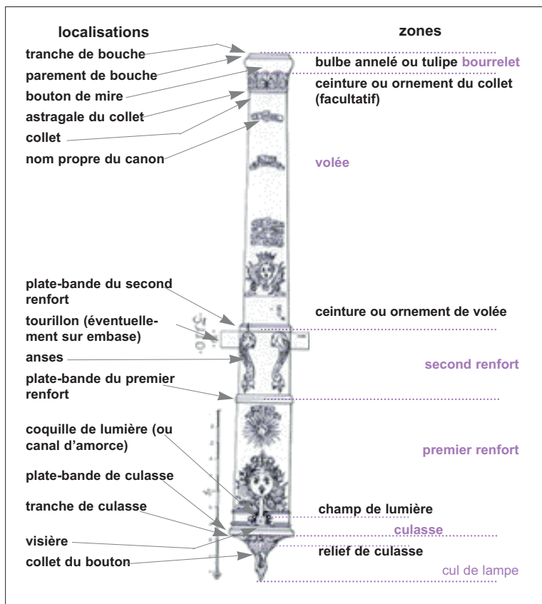
Morphologie d'un canon classique français. Dessin Claude Banar. © Paris, Musée de l'Armée/Drhap.
