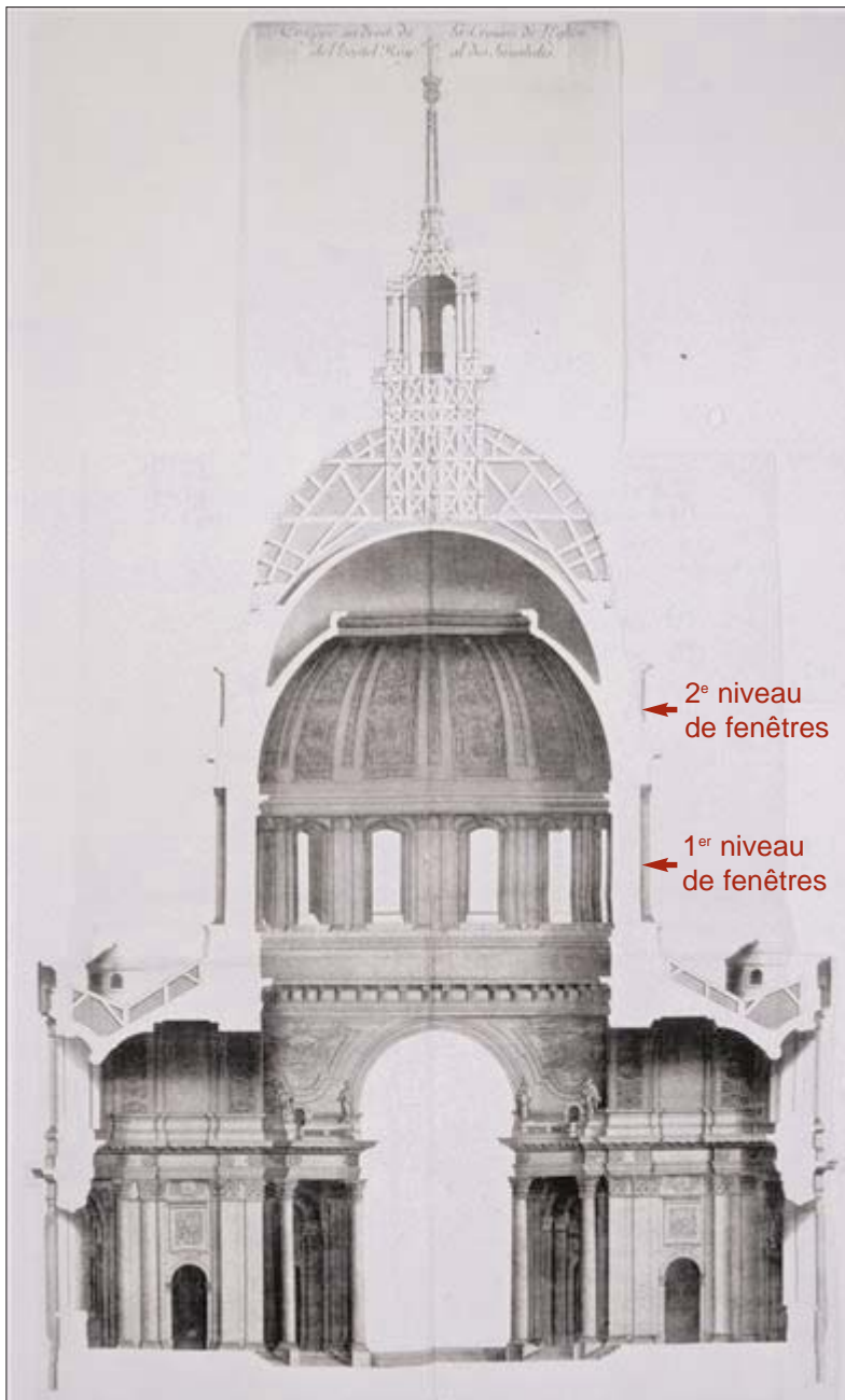
Coupe de l'église du Dôme. © Musée de l'Armée/RMN 07-503177.
